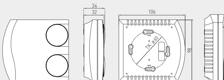
Plan coté
